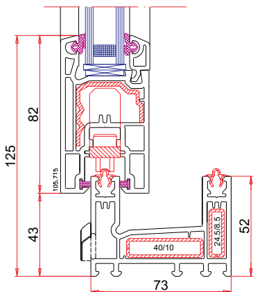
Detalle Corte
